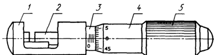
1 - корпус; 2 - микрометрический винт; 3 - стержень; 4 - барабан; 5 - трещотка (фрикцион)
