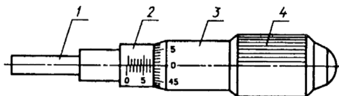
1 - микрометрический винт; 2 - стержень; 3 - барабан; 4 - трещотка (фрикцион)
