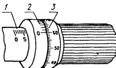
1 - стержень; 2 - нониус; 3 - барабан
